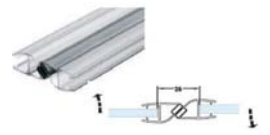
950.06.500 MAGNETIC SHOWER DOOR SEAL 180D, TRANSP. 1 pc
