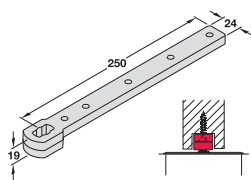
932.10.270 DOOR RAIL GEZE. Packing: 1 pc.
